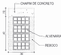
03 | CORTE AA ESC.: 1/15
