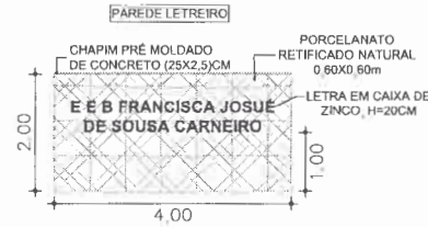
02 | DETALHE - PAREDE LETREIRO ESC.: 1/100
