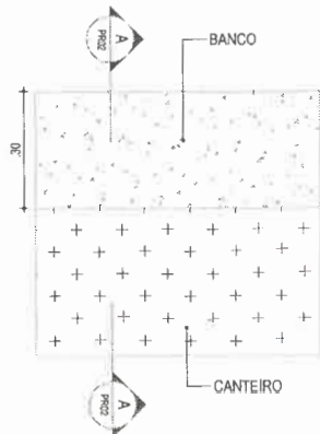
05 | PLANTA BAIXA - DETALHE CANTEIRO - BANCO ESC.: 1/10
