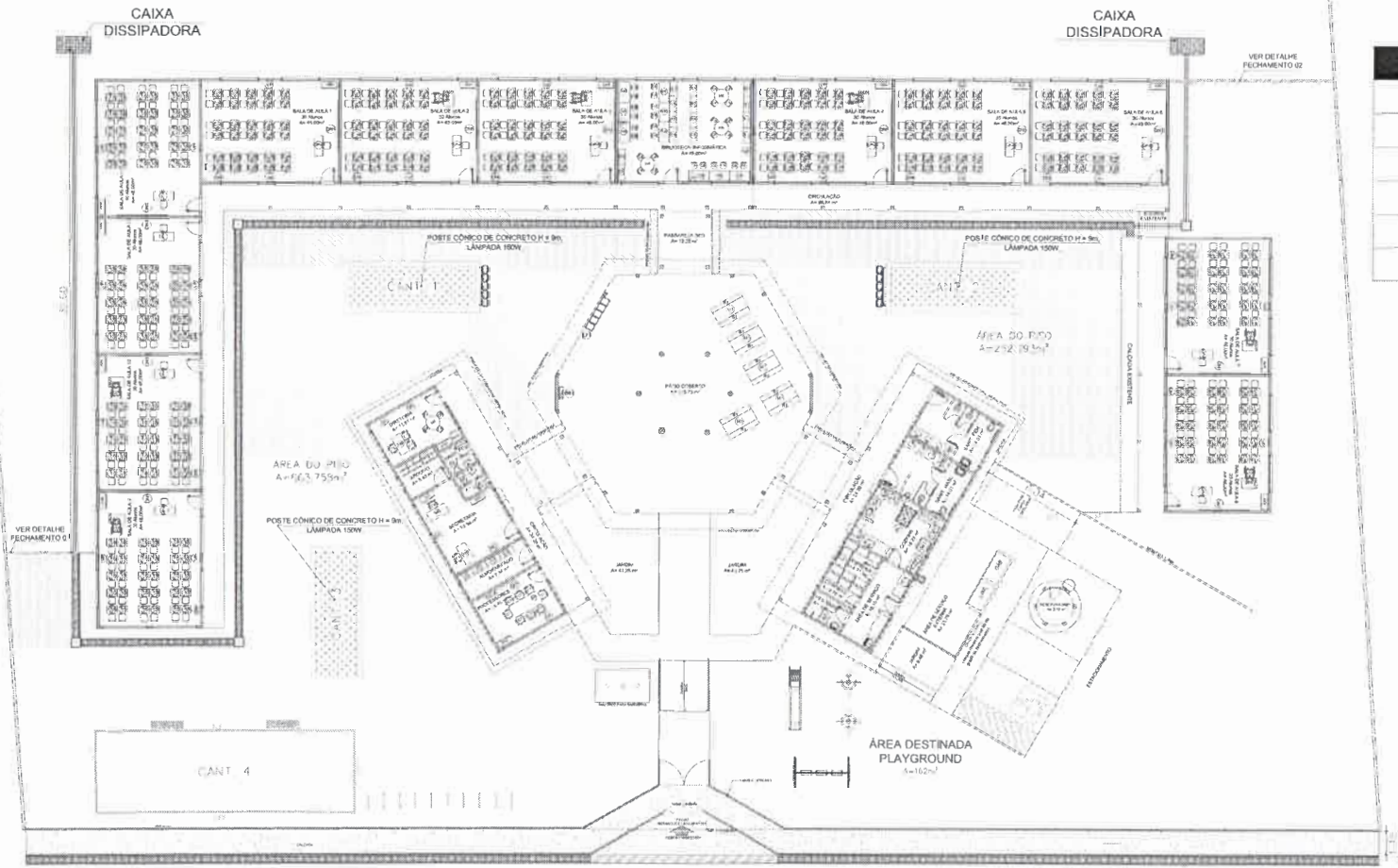
01 | PLANTA BAIXA EXTERNA - CALHA DE CONCRETO Esc. 1:200
