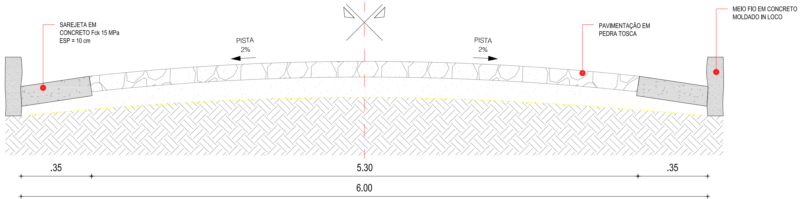
01 | SEÇÃO TIPO DE PAVIMENTAÇÃO ESC.: S/E
