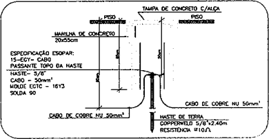
DETALHE DO ATERRAMENTO-ESC-1/25
