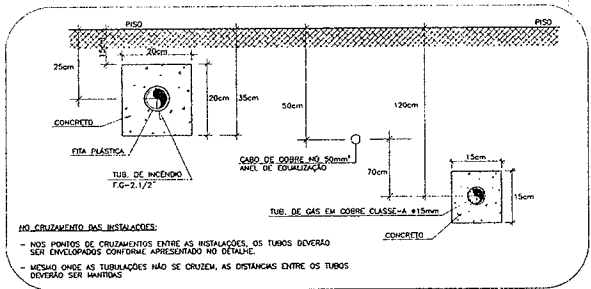
DETALHE DO CRUZAMENTO ENTRE AS TUBULAÇÕES-ESC-1/25
