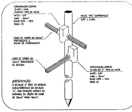
DETALHE "A" DA MASTE DE TERRA-ESC-1/25
