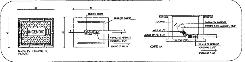
DETALHE DO HERANTE DE PASSO-ESC-1/25
