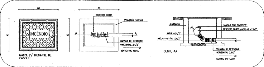
DETALHE DO HIRANTE DE PASSO-ESQ. 1/25
