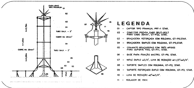
DETALHE DO PARA-RAIOS TIPO FRANKLIN-ESQ. 1/25
