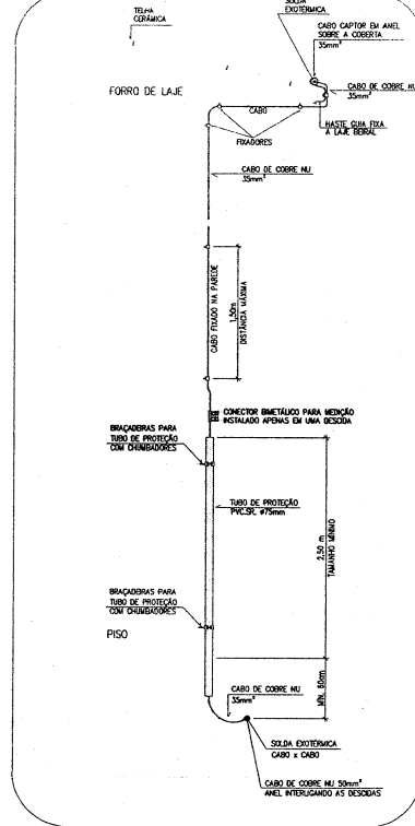
DETALHE ESQUEMÁTICO DA DESIDA DO SPMA-ESQ. 1/25
