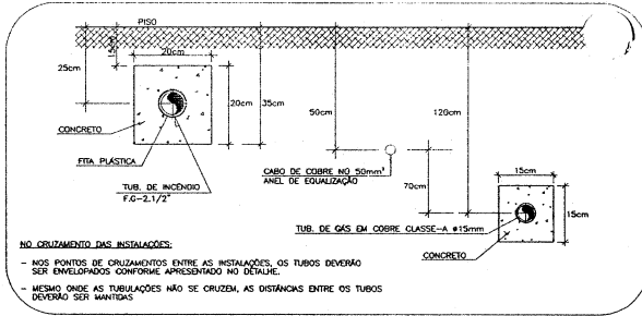
DETALHE DO ORIZAMENTO ENTRE AS TUBULAÇÕES-ESQ. 1/25
