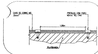
DETALHE DO CABO DE COBRE NA PLAINANDA-ESQ. 1/25
