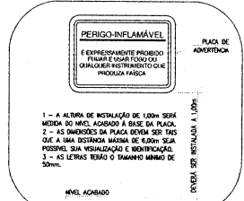
DETALHE PLACA DE ADERTECÇÃO-ESQ. 1/25
