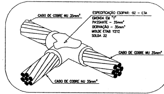
DETALHE "B"-SOLDA EXTERIORMENTE-ESQ. 1/25
