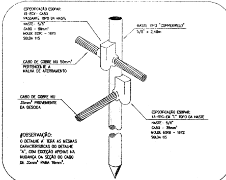
DETALHE "A"-DA MASTE DE TERRA-ESQ. 1/25
