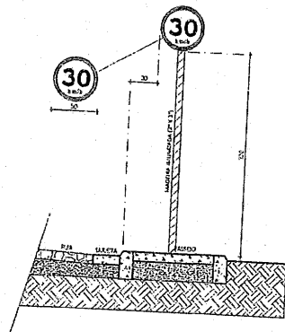
PLACA DE REGULAMENTAÇÃO TIPO R-19 (D=50cm)
