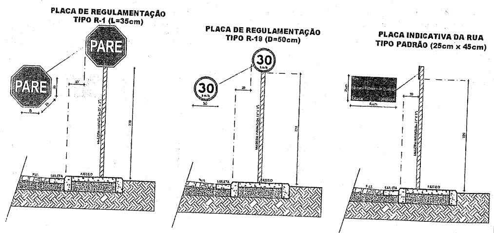
4 PERFIL TRANSVERSAL ESCALA 1:25
