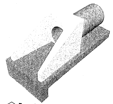
5 Bocas do Bueiro - Perspectiva ESCALA 1:20
