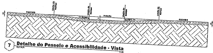
6 Detalhe do Passeio e Acessibilidade - Planta ESCALA 1:20
