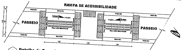
2 Detalhe do Passeio e Acessibilidade - Planta
