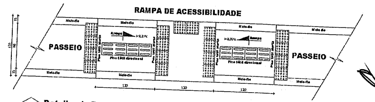
2 Detalhe do Passeio e Acessibilidade - Planta ESCALA 1:25
