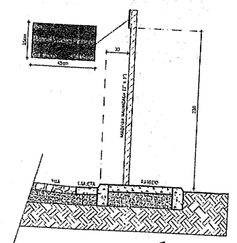
PLACA INDICATIVA DA RUA TIPO PADRÃO (25cm x 45cm)
